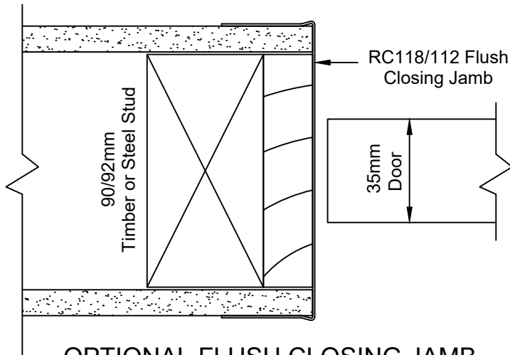
OPTIONAL FLUSH CLOSING JAMB
